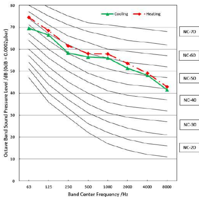
MUER-48-H14T-E
