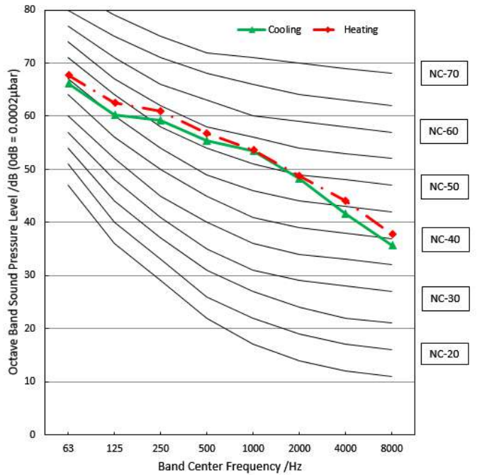
MUER-24-H14-E
