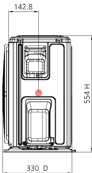
MUER-18-H14-E
