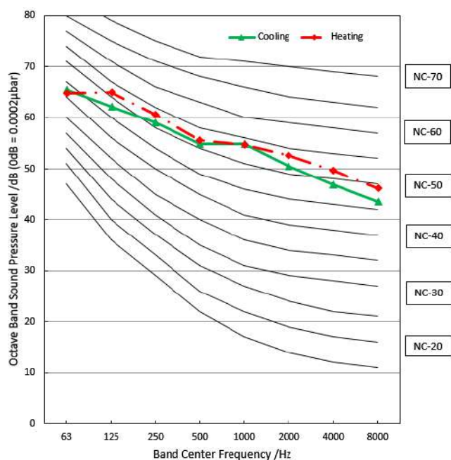
MUER-36-H14-E
