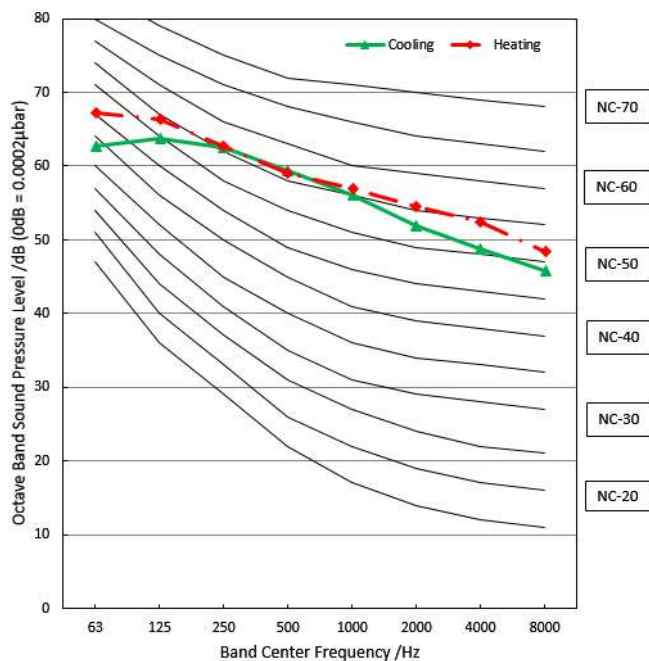
MUER-36-H14-E
