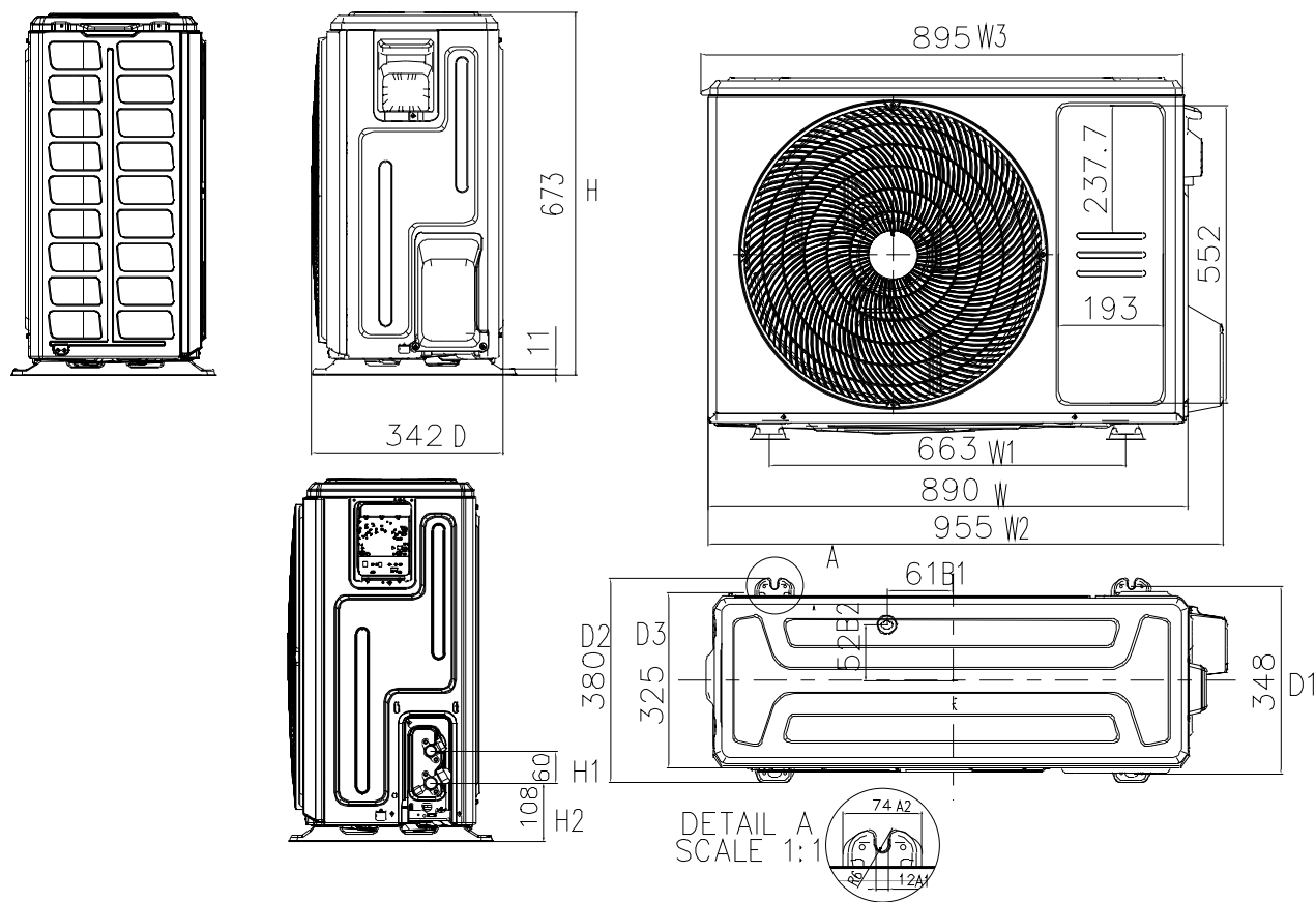
MUER-24-H14-E
