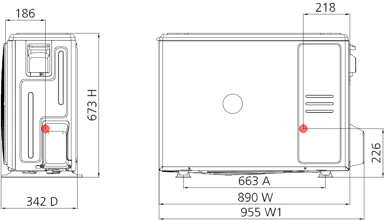
MUER-24-H14-E
