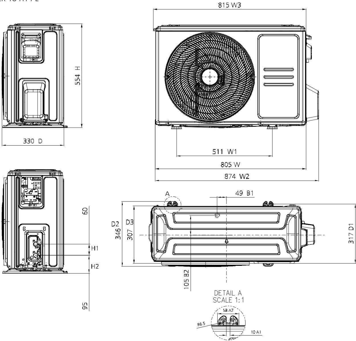
MUER-18-H14-E
