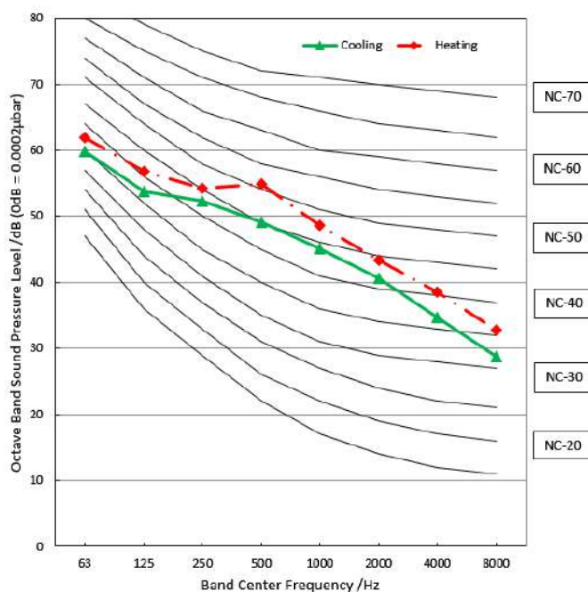
MUER-18-H14-E
