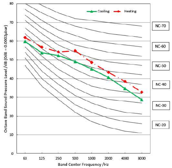
MUER-24-H14-E
