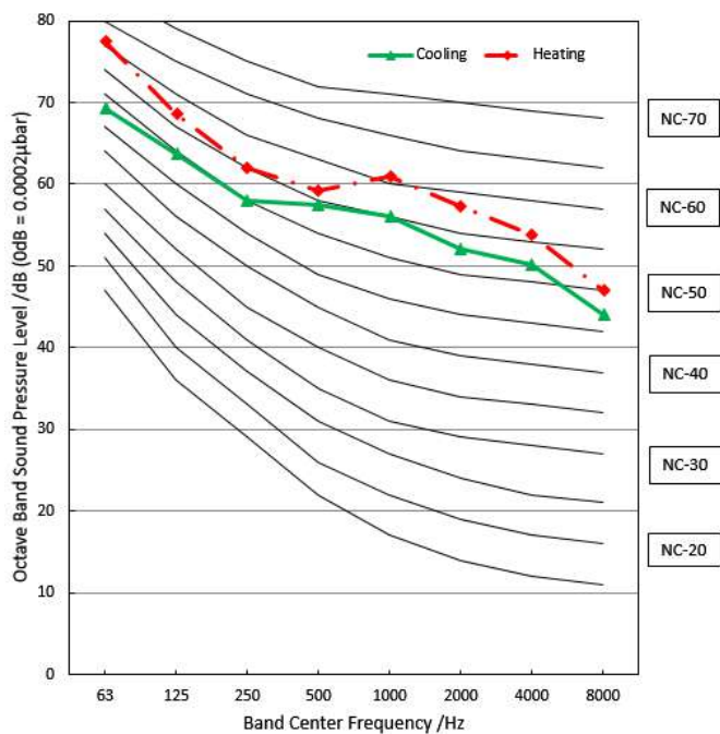
MUER-60-H14T-E
