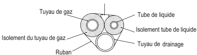
Câblage d'interconnexion
