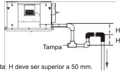
Figura 5.3 Esquema do sifão de armazenamento de água
