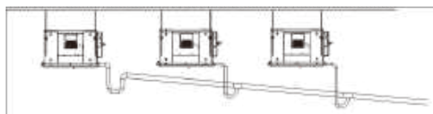
Inclinação para baixo de 1/100 ou mais
