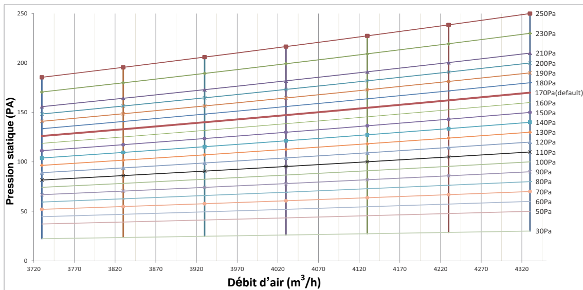
Illustr. 6.2 : Modèles 200 / 250 / 280
