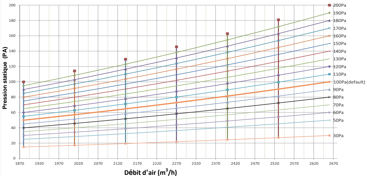
Illustr. 6.2 : Modèles 200 / 250 / 280
