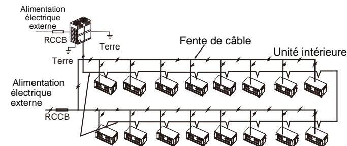
Câble de communication entre l'unité intérieure et l'unité extérieure
