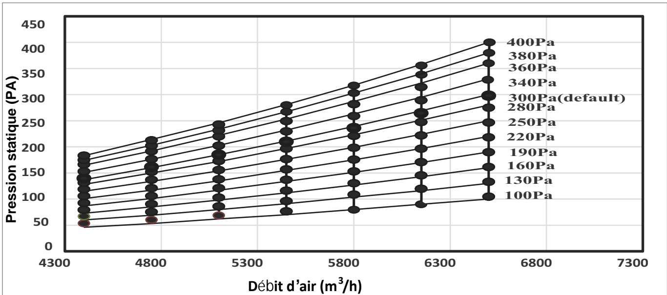
Illustr. 6.4 : Modèle 560
