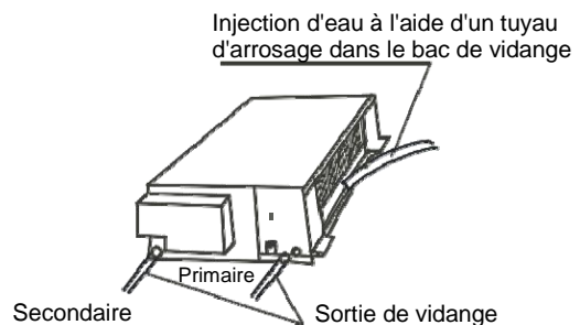
Figure 5.4 Vérification de l'évacuation de l'eau
