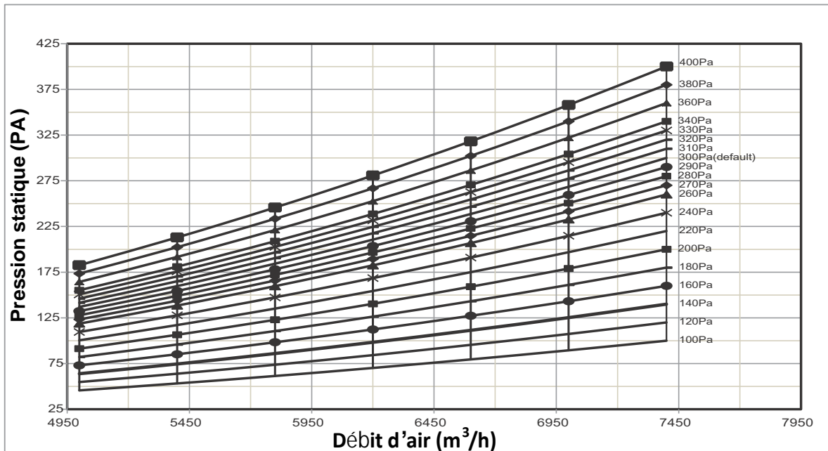
Illustr. 6.4 : Modèle 560
