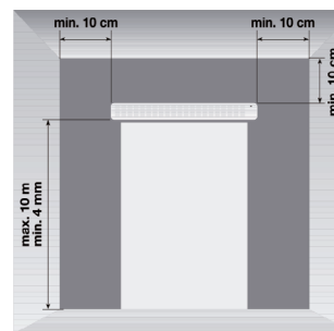
Hauteur d'installation.
