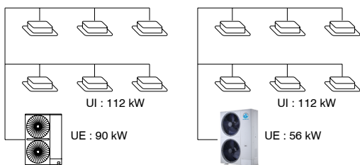
Système VRF traditionnel
