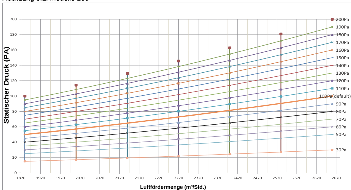
Abbildung 6.2: Modelle 200/ 250/ 280
