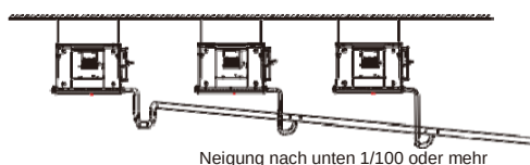
Abbildung 5.2a (ohne Wasserpumpe)
