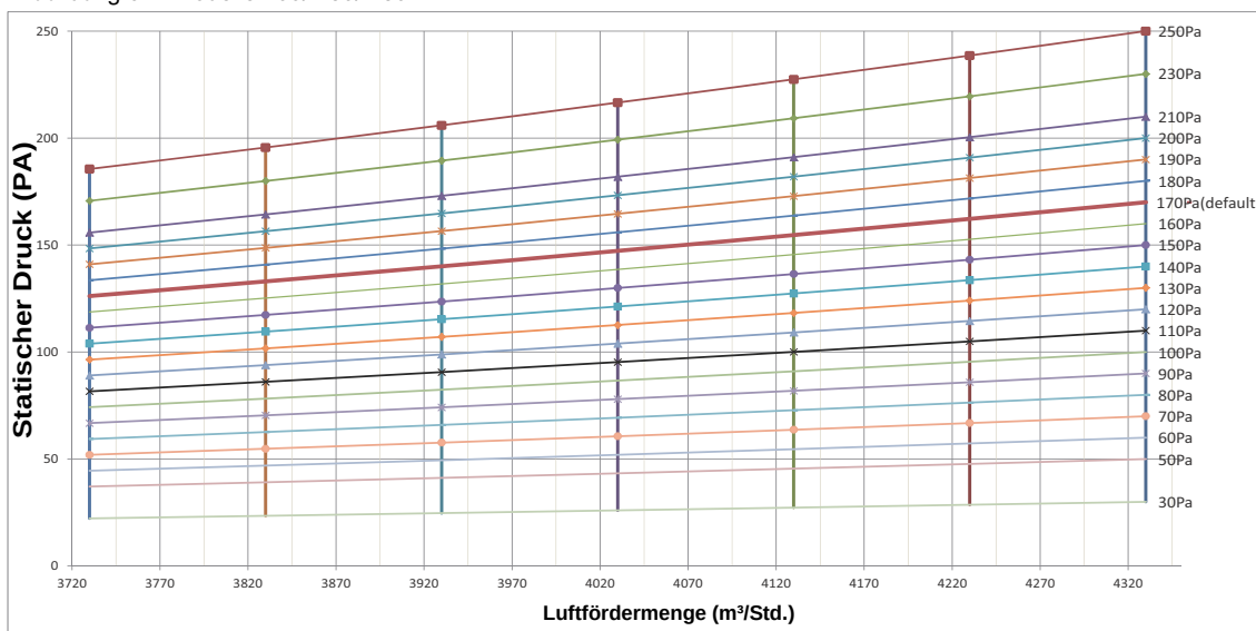
Abbildung 6.2: Modelle 200/ 250/ 280
