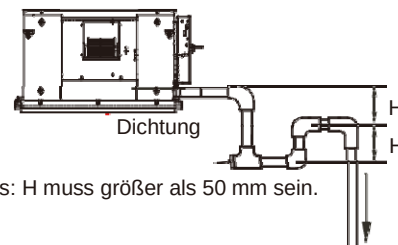
Abbildung 5.3 Schema des Wasserspeichersiphons
