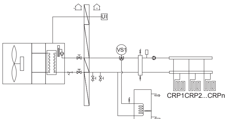
Schema dell'impianto 2
