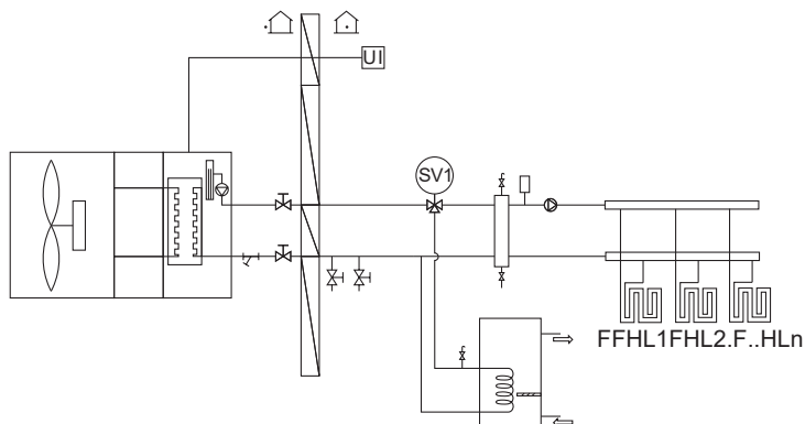
Układ systemu 2
