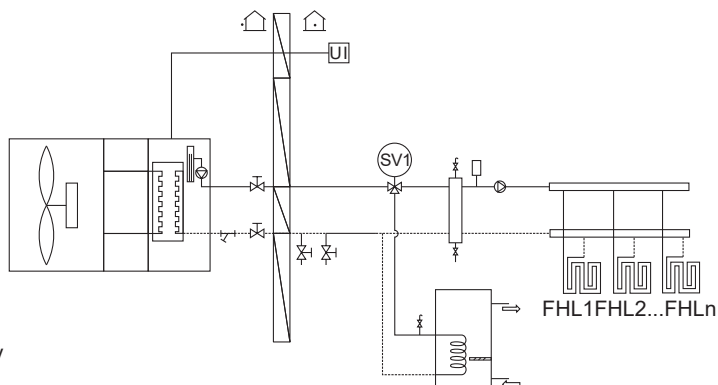
Układ systemu 1
