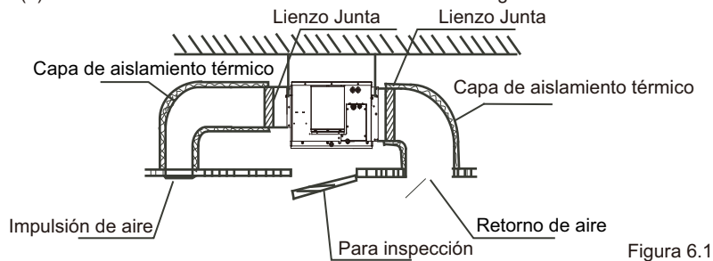
Figura 6.1: Modelo 160
