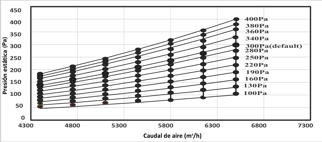
Figura 6.4: Modelo 560
