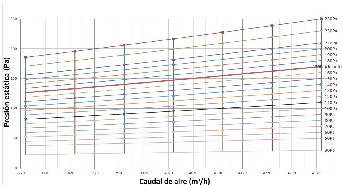
Figura 6.2: Modelos 200 / 250 / 280
