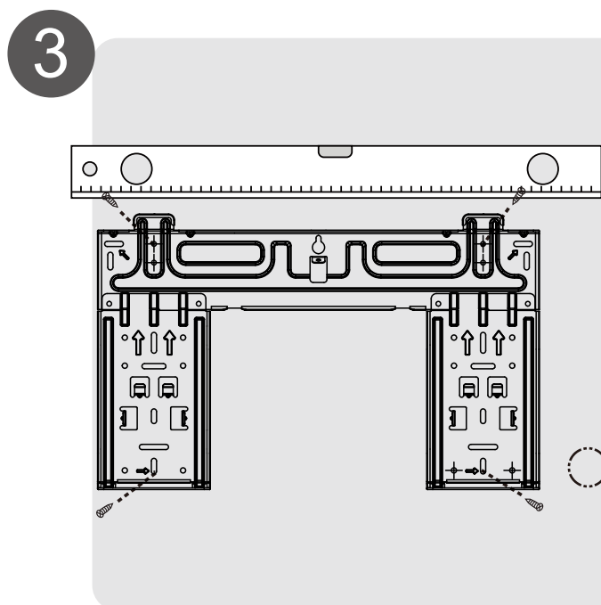
Fije la placa de montaje (Pág. 15)
