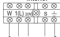
Terminais da unidade interior
