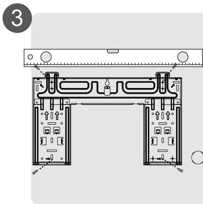
Fije la placa de montaje
