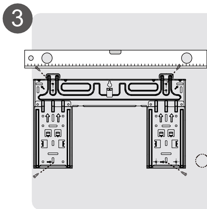
Befestigen Sie die Montageplatte
