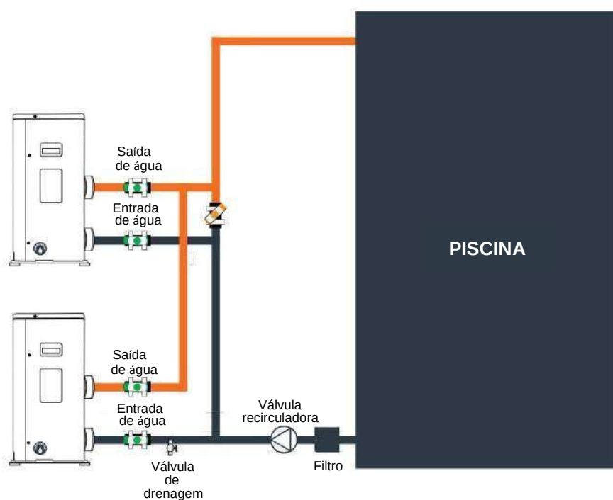
Diagrama de instalação em paralelo
