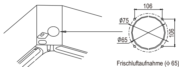
Frischluftaufnahme (φ 65)
