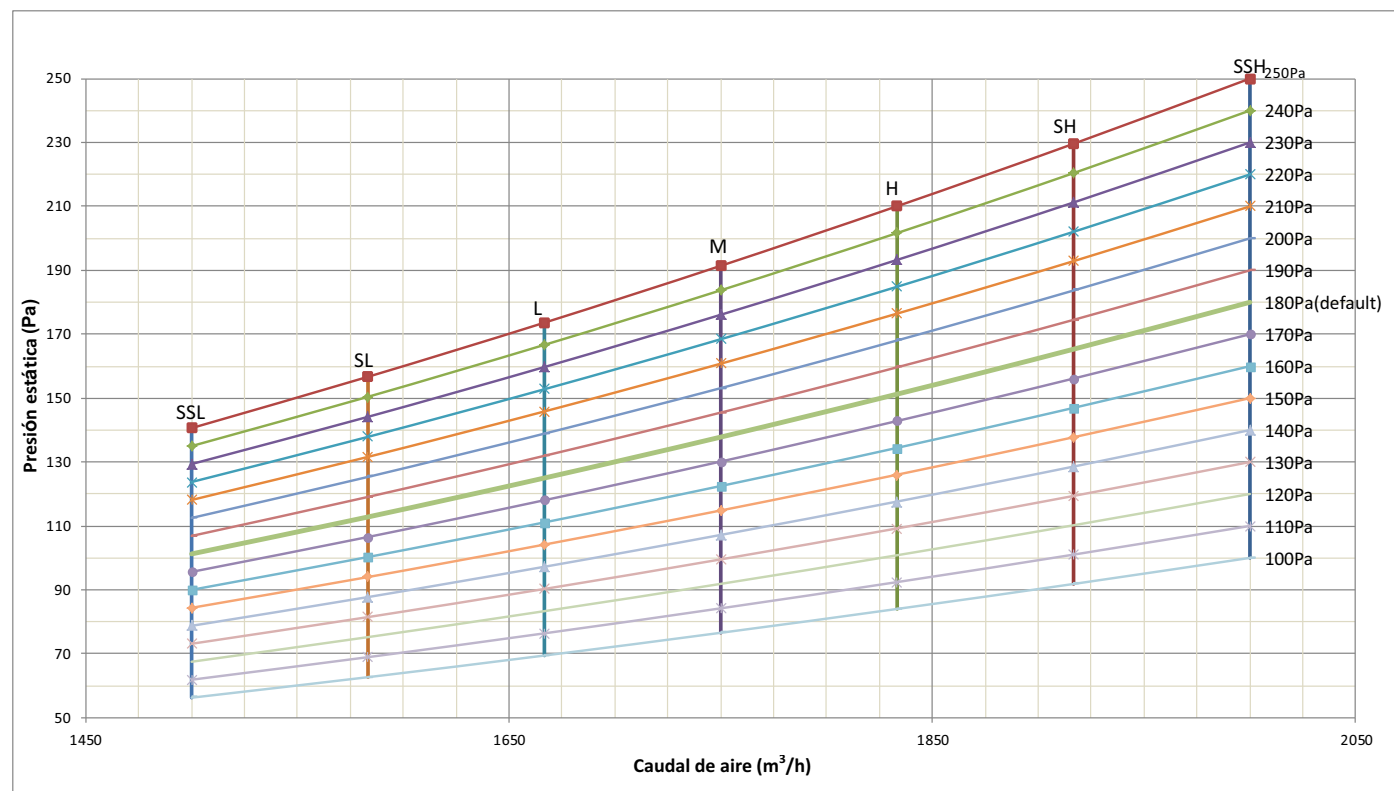
Figura 6.1: Modelos 125 / 140
