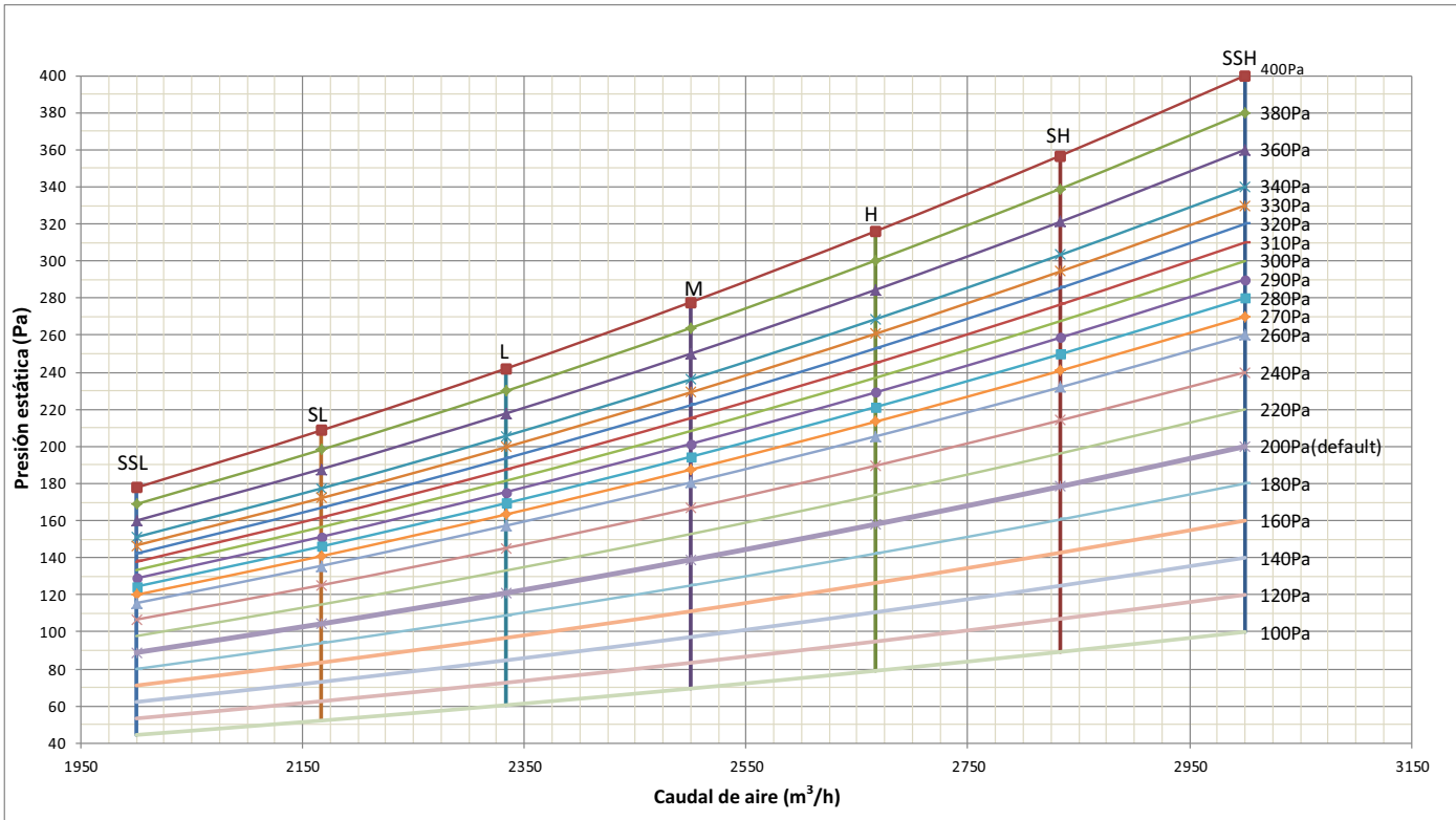
Figura 6.2: Modelos 200 / 250 / 280
