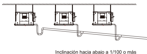
Figura 5.2a (sin bomba de agua)
