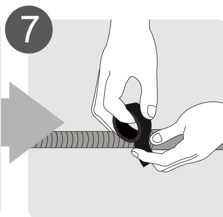
7 Preparación de la tubería de drenaje (pág. 14)
