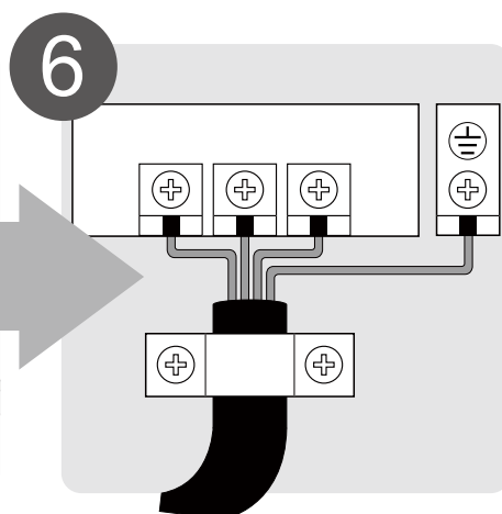
6 Conexión del cableado (pág. 17)
