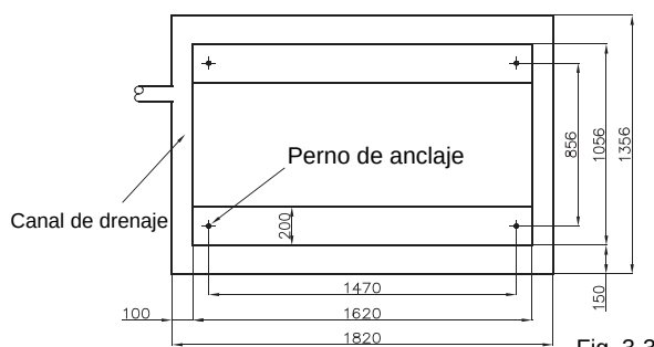
Diagrama de instalación de las dimensiones de la unidad
