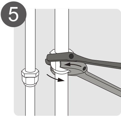
5 Tubería de conexión (pág. 25)
