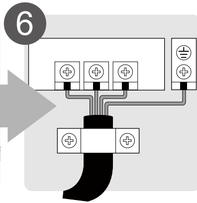
6 Conexión del cableado (pág. 17)
