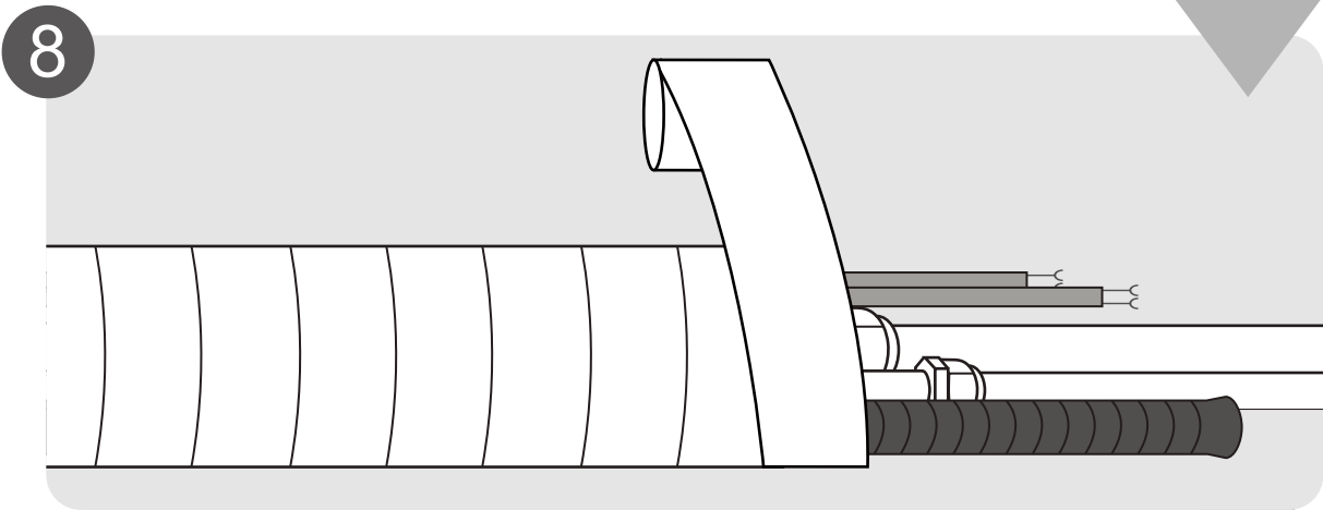
8 Envolver tuberías y cables (pág.18)
