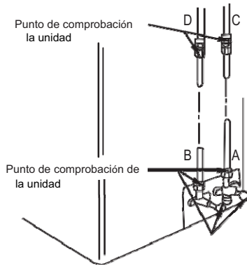
A. Válvula de cierre en baja B. Válvula de cierre en alta C, D. Juntas de la tubería de conexión a la unidad interior.
