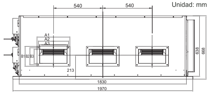
Vista frontal (Impulsión de aire)
