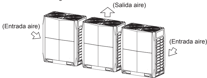
Espacio de servicio y funcionamiento Fig.4-7
