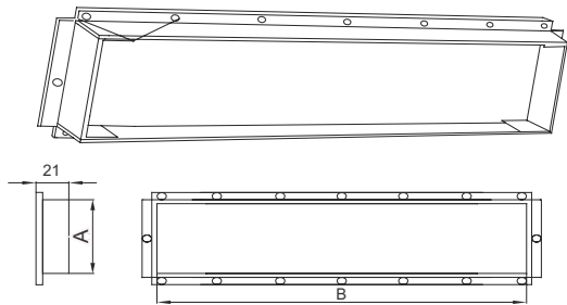
Fig.34 Suministro de salida de aire
