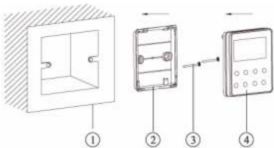
Fig.26 Piezas estándar del termostato
