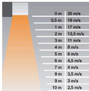
Distancia/velocidad aire.
