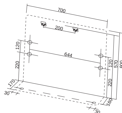
Diagrama de ganchos de montaje
