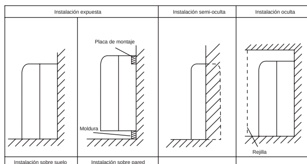
Ubicación para fijar el panel de montaje
