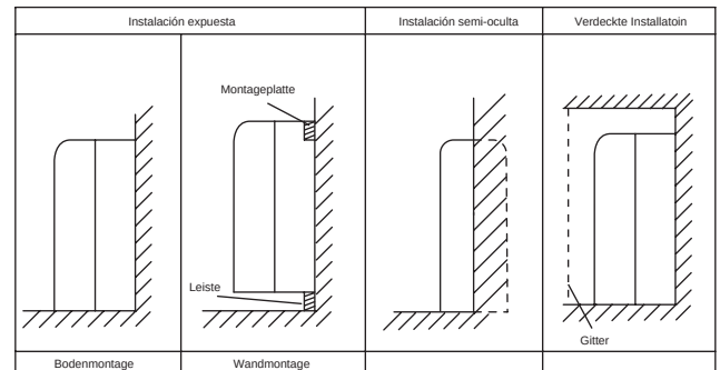
Lage zur Befestigung der Montageplatte
