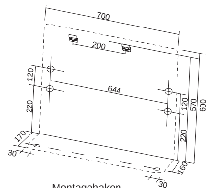
Montagehaken
