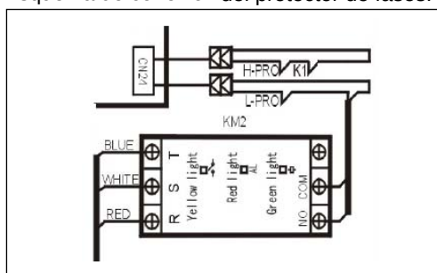
Esquema de conexión del protector de fases:
